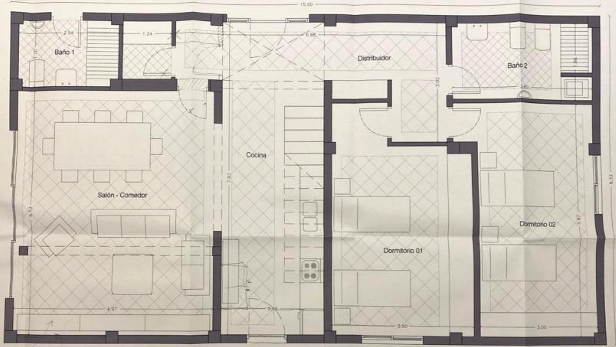
ESTADO REFORMADO 01 PLANTA BAJA
